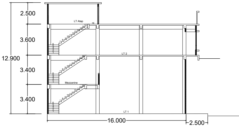
Potongan ruko
