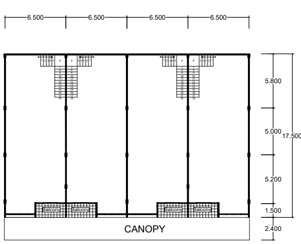
Lantai 2
